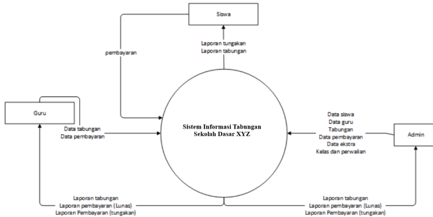
Gambar 3. Diagram Konteks
